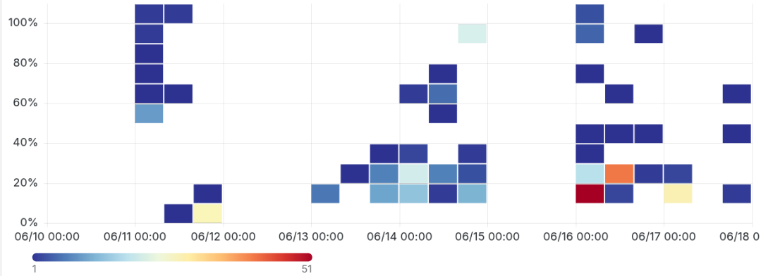
Mapa de Calor - Humedad del Suelo (Area 1)
